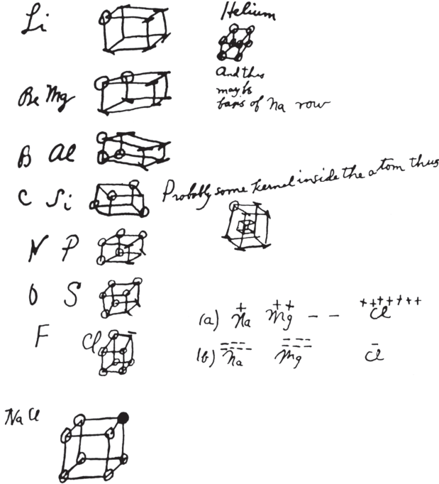
شكل ٧-٢: مخطّط لويس عن «المكعبات» الذرية.
