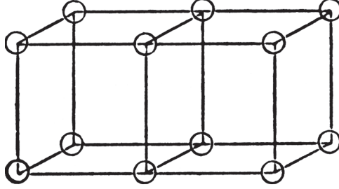
شكل ٧-٣: تصوّر لويس لرابطة ثنائية بين ذرتين.
